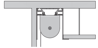
Einbau in abgehängte Decke Wand-/ Fassadenbündig (MP-80-V3)
