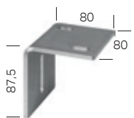
Montagewinkel für MP-80 V2A inkl. Befestigungsschrauben
