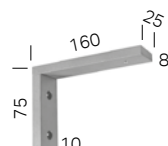
Wandträger 16 cm
