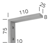
Wandträger 11 cm
