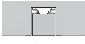
Einbau in Decke (MP-80-V1)
