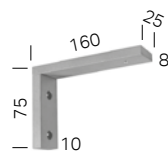
Wandträger 16 cm
