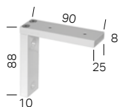
Wandträger 9 cm
