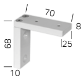
Wandträger 7 cm
