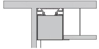
Einbau in abgehängte Decke Wand-/ Fassadenbündig (MP-80-V3)
