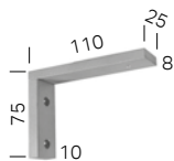
Wandträger 11 cm
