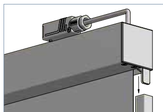
E-63-A Aufständering
