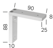
Wandträger 9 cm Behang vorne abrollend
