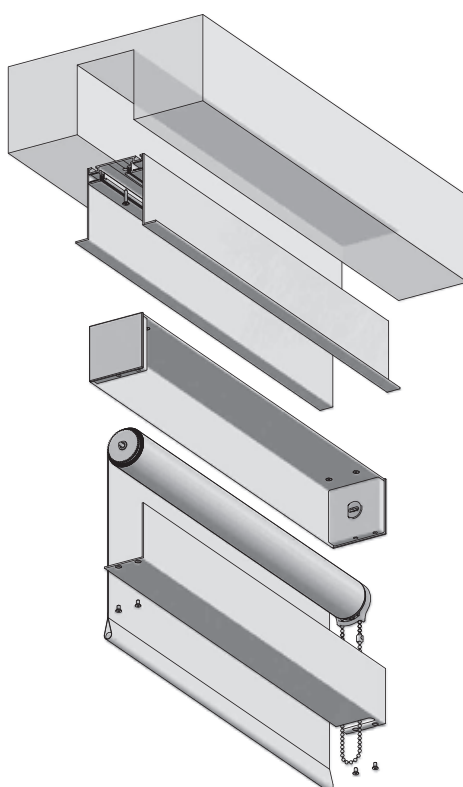
Funktionsweise Einbau
