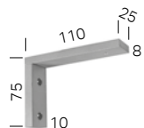
Wandträger 11 cm
